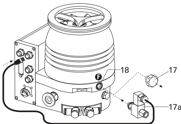
Fig. 8: Raccordement de la vanne de remise à l'air
