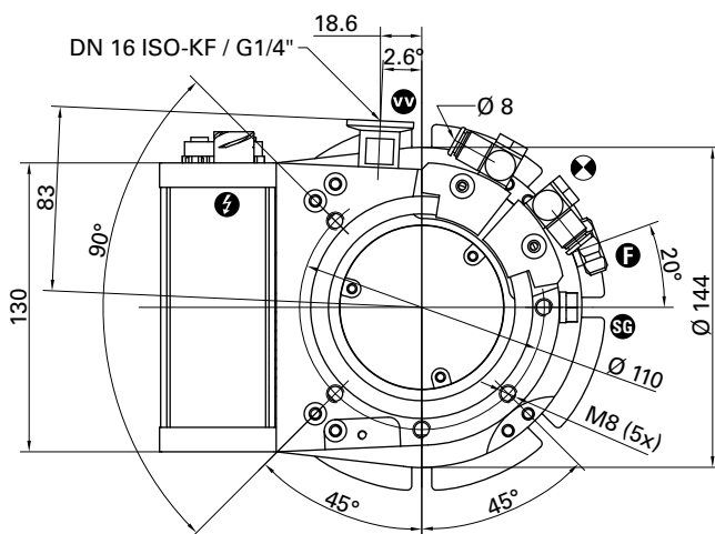
Fig. 17: HiPace 300 P, DN 100 ISO-F
