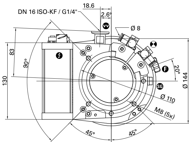
Fig. 16: HiPace 300 P, DN 100 CF-F
