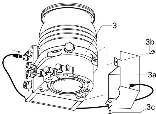
Fig. 7: Raccordement du refroidissement par air
